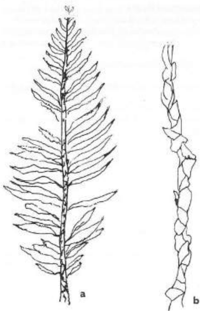
Fig. 17- Sequoia langsdorffii (a-x 1,5; b-x 4,5)
