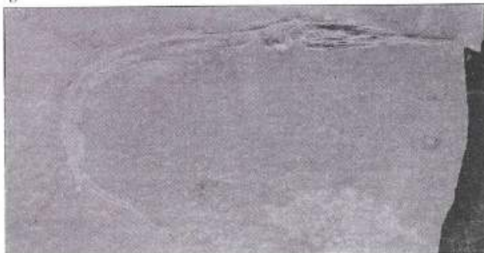
Fig. 83- Systolichthys catalaunicus (a - original de BELTAN, 1972) (b - x 0,4) Alcover / Mont-Ral
