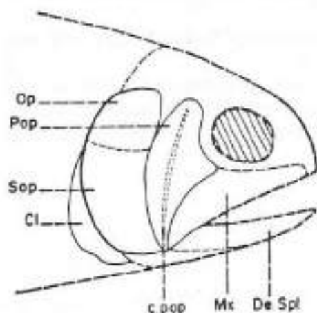
Fig. 81- Meidiichthys sp. (original de BELTAN, 1972) Alcover / Mont-Ral
