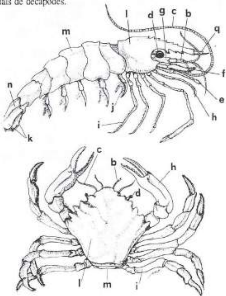
Fig. 57- Morfologia dels decàpodes més freqüents:
