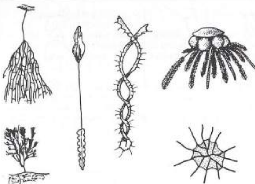
Fig. 69- Diferents tipus de colònies de graptòlits (dibuix: Jordi Miró)
