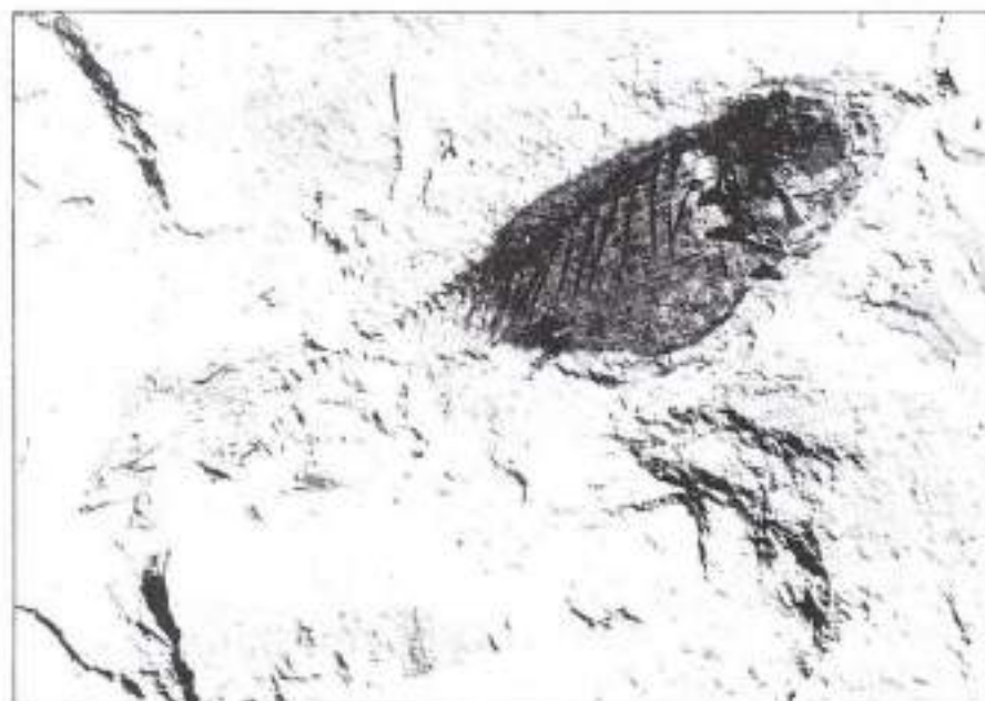
Fig. 89- Prolebias catalaunicus . Sarrià a) x 2,5 (dibuix: J. GAUDANT, 1982) b) x 2,5 (Foto: Ferrn Civil)
