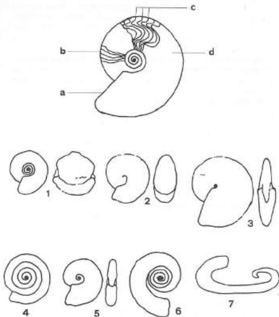
Fig. 51- Morfologia típica d'un cefalòpode:
