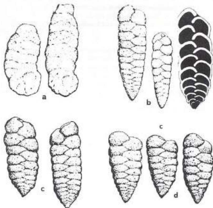
Fig. 12 - Foraminífers textularins: a) Ammobaculites hockleyensis b) Textularia recta c) Textularia elegans d) Textularia budensis . Pontils (extret de G. COLOM, 1972)
