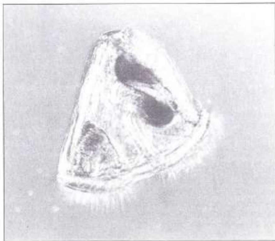
Fig. 38 A- Larva cífonaute de briozou actual (x 120)
