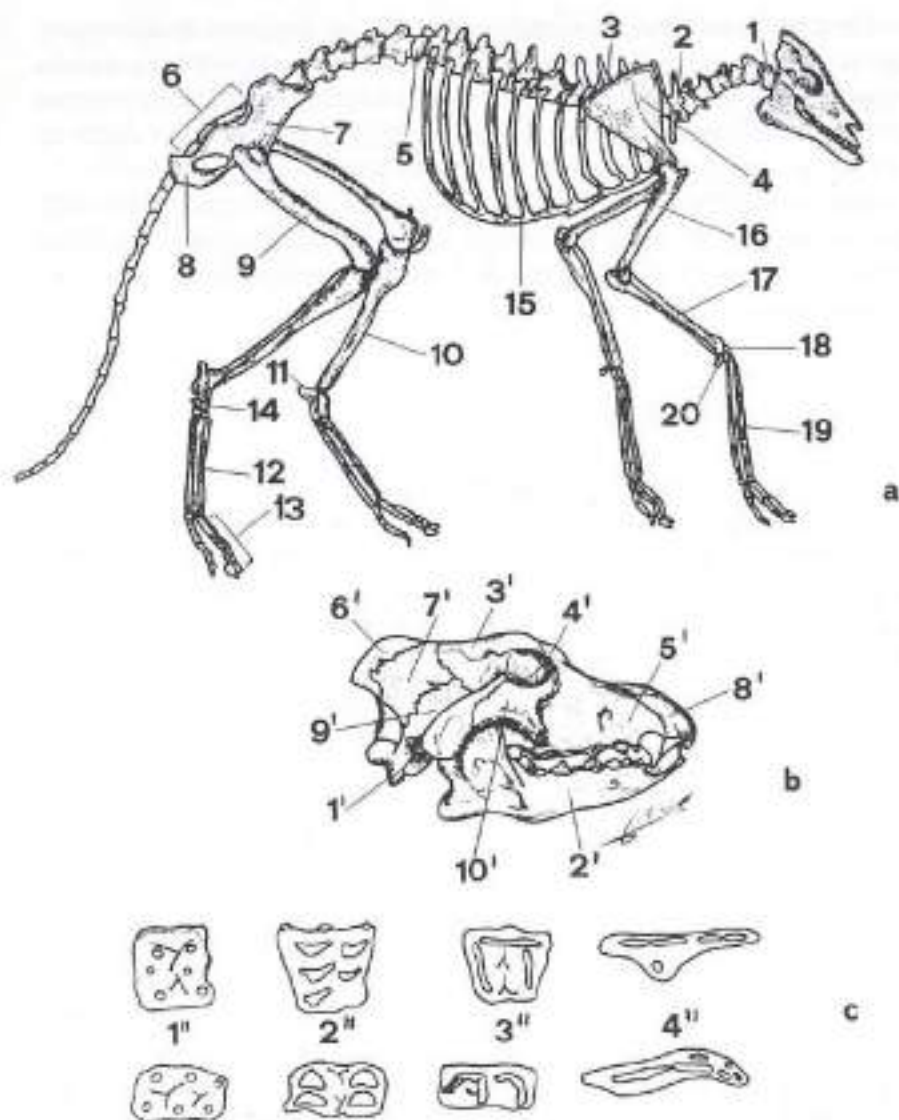
Fig. 94- Morfologia de l'esquelet dels mamífers:
