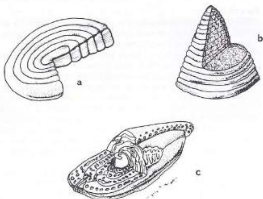
Fig. 11 - Forma de la closca dels foraminífers més freqüents, amb seccions on es veuen les cambres.
