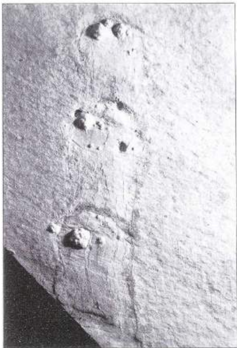
Fig. 100- Equisetites sp. (x 0,8) El Pintell
