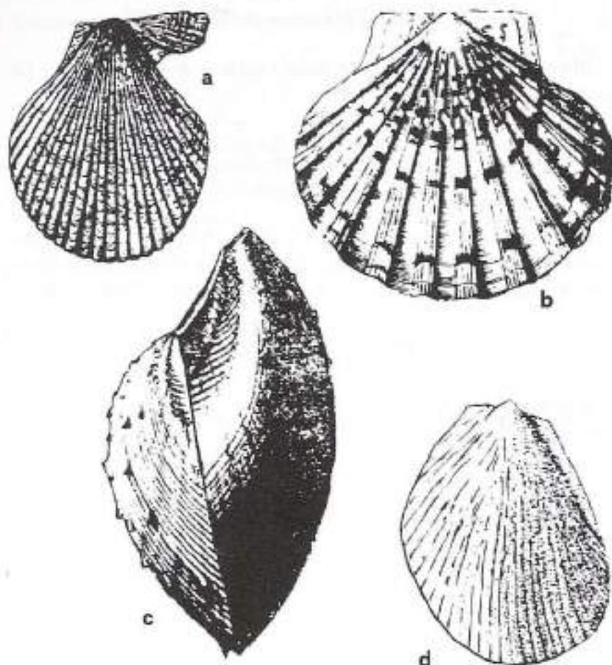
Fig. 49- Bivalves pteriomorfs cocens:
