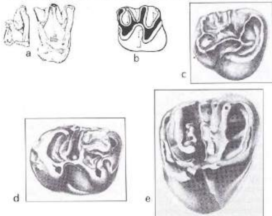
Fig. 95- Quiròpters i rosegadors (molars):
