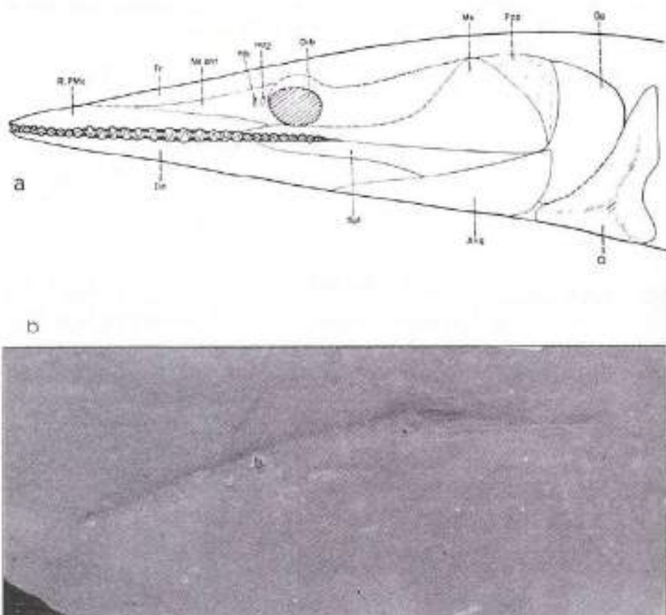
Fig. 82- Brevisaurichthys osseus (a - original de BELTAN, 1972) (b - x 0,5) Alcover / Mont-Ral
