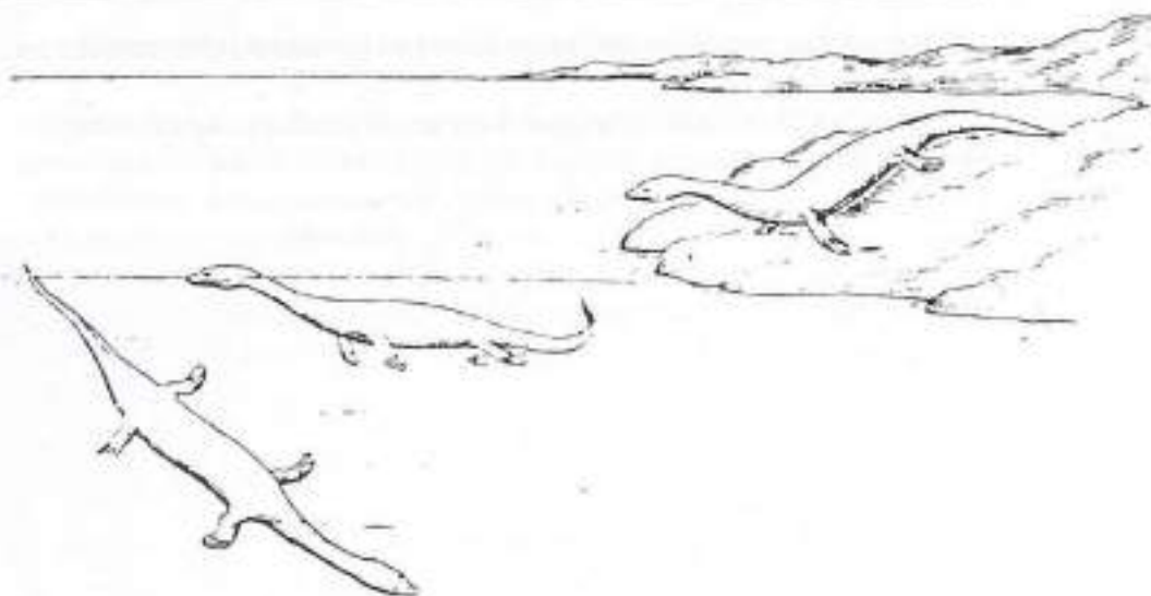
Fig. 91.- Notosàurids al seu hàbitat suposat (segons W. Erhardt)
