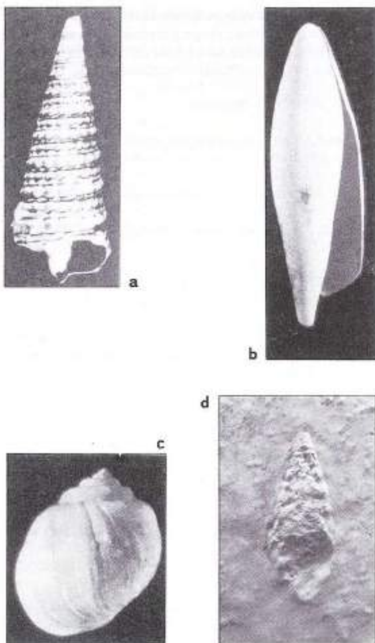
Fig. 45- a) Potamidés sp. (x 1,5) b) Terebellium sp. (x 1,5) c) Ampullina sp. (x 1,5) d) Loxonema sp. (x 1) Alcover / Mont-Ral (extret: a de LÓPEZ, 1987 b i c de GOMEZ ALBA, 1989)
