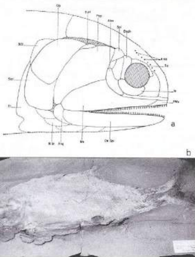
Fig. 79- Perleidus giganteus (a - original de BELTAN, 1972) (b - x 0,12) Alcover / Mont-Ral
