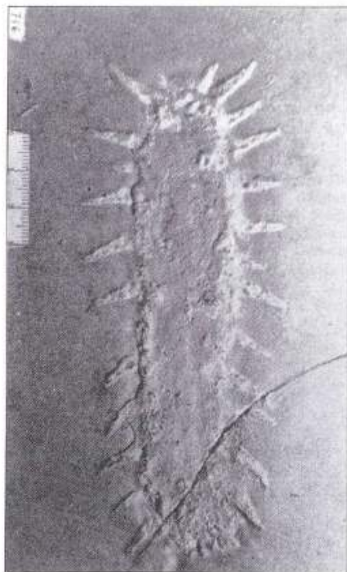
Fig. 66- Oneirophantites tarraconensis (x 1) Alcober / Mont-Ral
