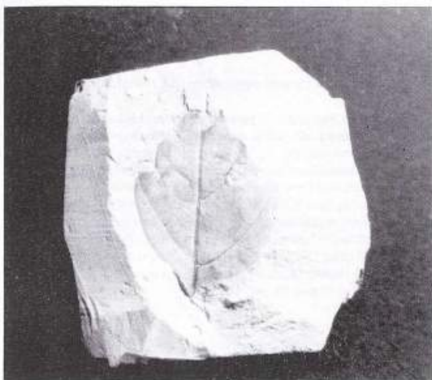
Fig. 28- Rhus phryrae (x 2) Sarra (Foto: Fermí Civit)
