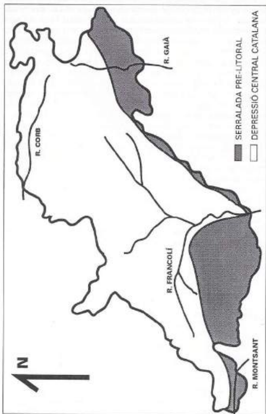
Fig 2. Mapu de les unitats fisiogràfiques al sector de la Conca
