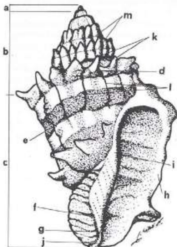
Fig. 41- Morfologia típica de la conquilla d'un gasteròpode: a) protoconquilla b) espira c) darrera volta d) sutura e) callositat columel·lar f) solc umbilical g) obertura h) llavi palatal i) llavi parietal j) canal sifonal k) espines l) còstules axials ll) cordons espirals (dibuix: Jordi Miró)
