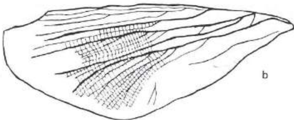
Fig. 60- Montralia mülleri (a - x 0,8) (b - x 1,5) (dibuix: VIA i CALZADA, 1987)
