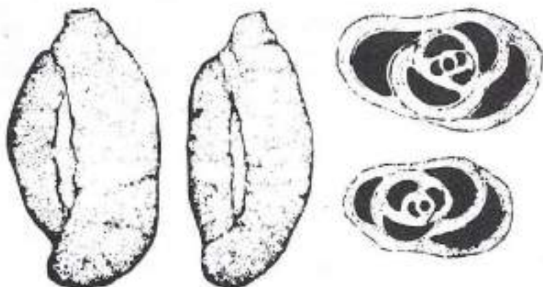
Fig. 13 - Foraminífers miliolins Triloculina mollis , Castell de Queralt (extret de G. Colom, 1972)
