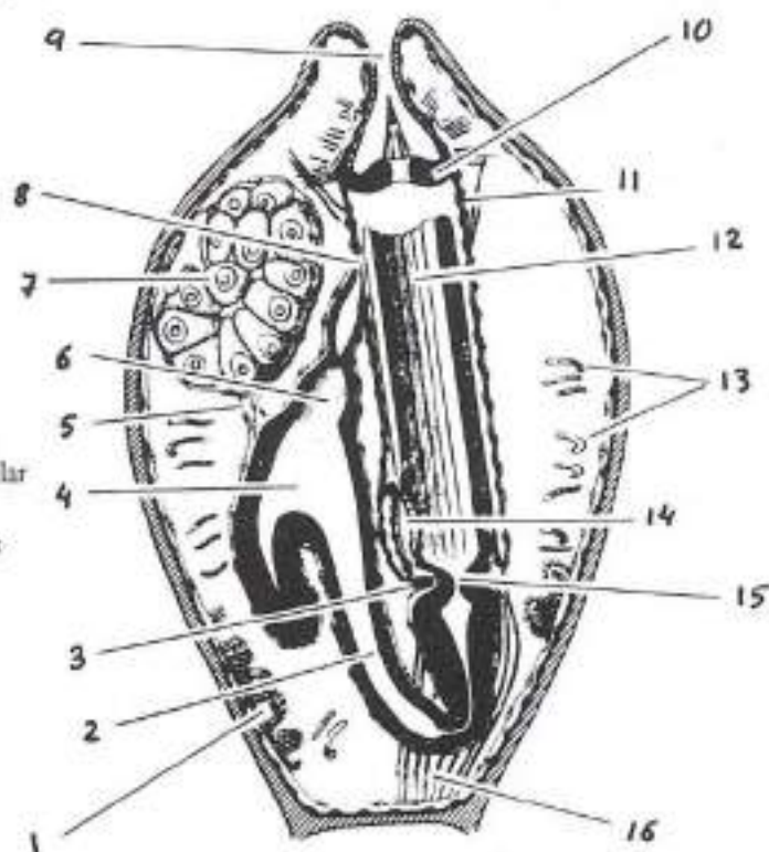
Fig. 36- Morfologia típica d'un zooïde de briozou.
