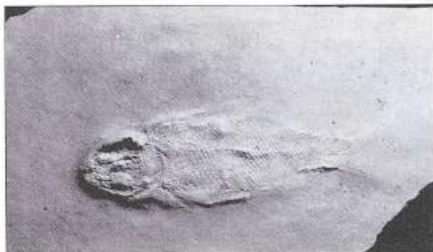
Fig. 78- Perleidus viai (a - original de BELTAN, 1972) (b - x 0,8) Alcover / Mont-Ral
