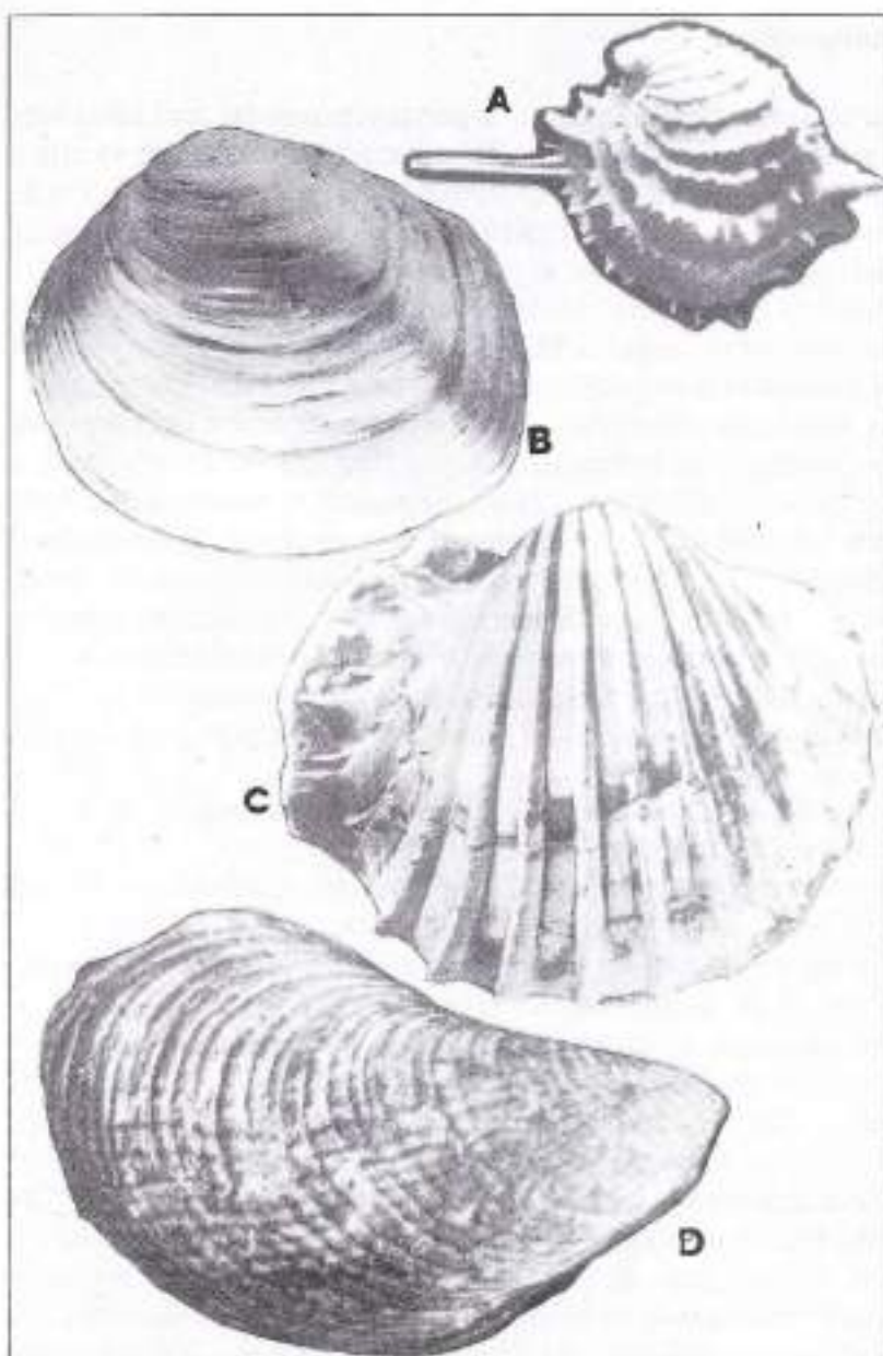
Fig. 50. Bivalves heterodonts i anormalodèsimats:
