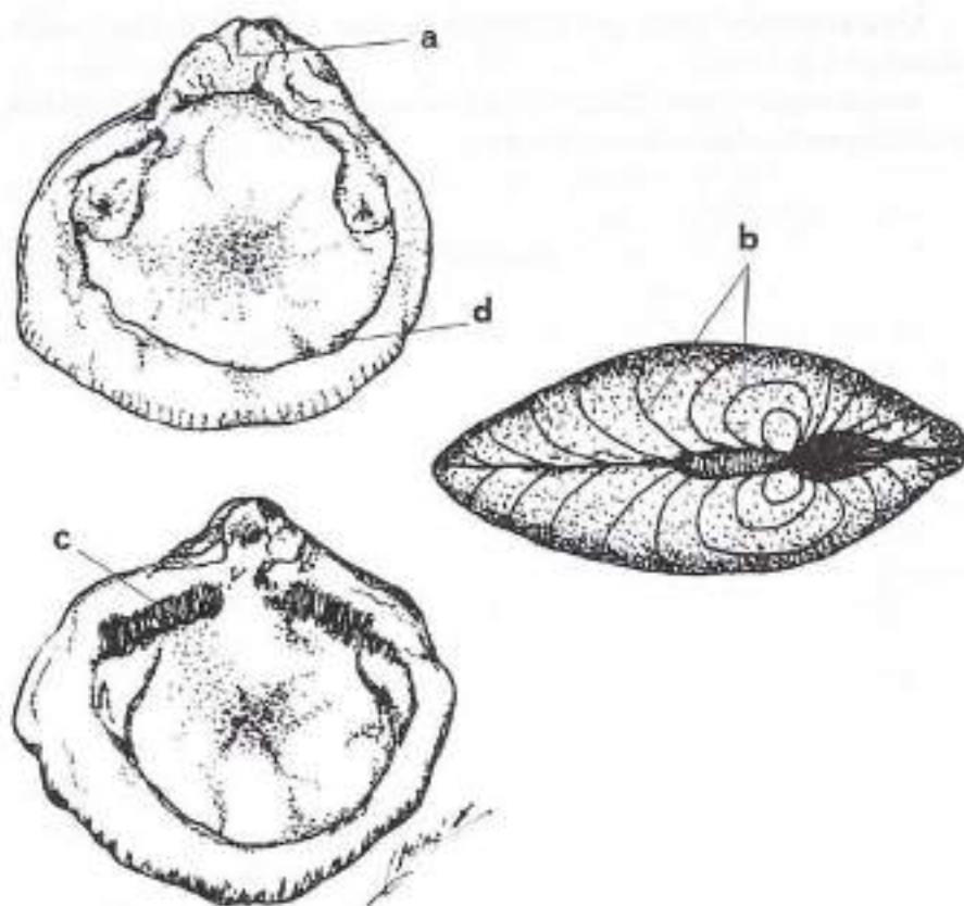
Fig. 47- Conquilla típica dels bivalves: a) umbe, b) línies de creixement, c) xarnera, d) línia palcal (dibuix: Jordi Miró)
