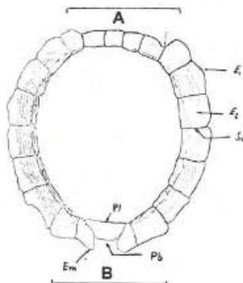
Fig. 9- Morfologia d'un girogonit de caròfit:
