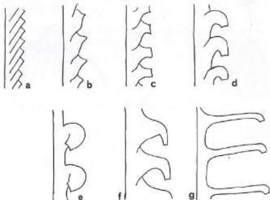
Fig. 70- Tipus de teques d'un graptòlit:
