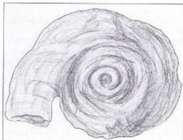
Fig. 35- Rotularia spirulaea (x 5) (dibuix: Jordi Miró)
