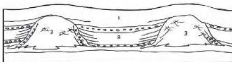
Fig. 97- La pedra d'Alcover es va omplir les cubetes dels esculls de la Riba. 1) tram superior de la pedra d'Alcover, 2) tram inferior de la pedra d'Alcover, 3) esculls de la Riba. (original de F. Calvet, reelaborat per l'autor)
