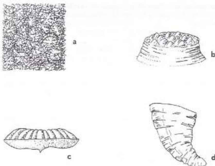
Fig. 31- Formes de cnidaris presents a la Conca:
